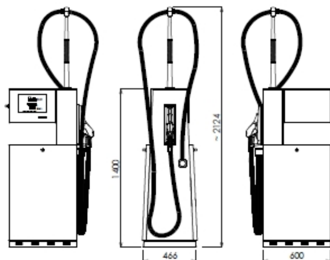
BMP511.SR/AdB-HS
