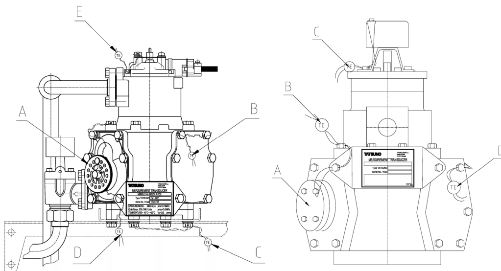
Obrázek 95 – Pístové měřiče PHM (typ FM-1007) a LPG (typ MP-02524 a FM-1029), A=kalibrační kolečko
