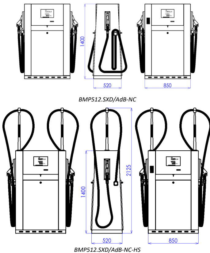
Obrázek 11 - Standardní modely stojanů SHARK ECONOMY /ADB (nesoučasná čerpání „-NC“)
