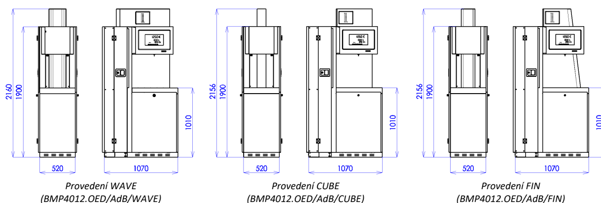
Obrázek 21 – Designové varianty stojanu OCEAN EURO /ADB
