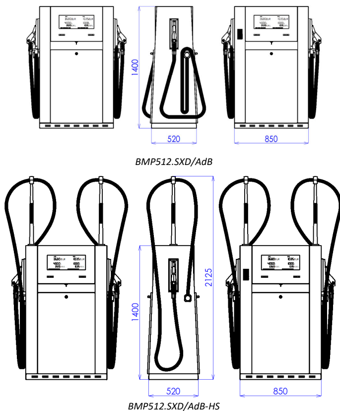
Obrázek 10 - Standardních modely stojanů SHARK ECONOMY /ADB (dvě současná čerpání)
