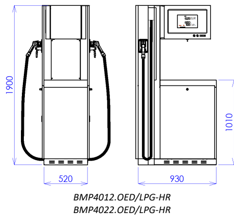
Image 6 - Aperçu des modèles standards d'appareils distributeurs OCEAN EURO GPL avec
