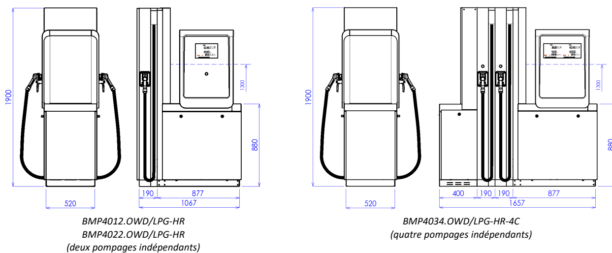
Image 8 – Modèle standard d'appareil distributeur OCEAN TOWER GPL avec enrouleurs de flexibles de distribution
