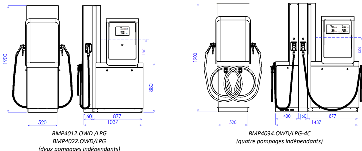
Image 7 – Modèles standards de l'appareil distributeur OCEAN TOWER GPL avec flexibles librement suspendus
