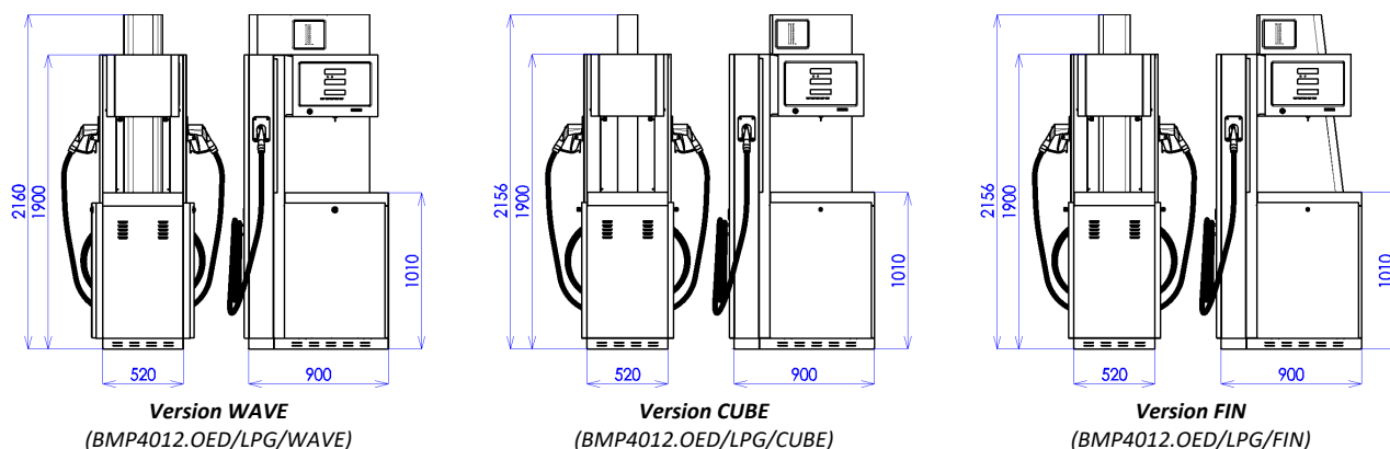
Image 4 – Variantes de design des modèles d'appareils distributeurs OCEAN EURO GPL
