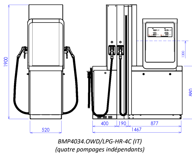
Image 9 – Variante italienne spéciale de l'appareil distributeur OCEAN TOWER GPL avec deux enrouleurs de flexibles de distribution et deux flexibles librement suspendus (pour une plus grande portée du pistolet de distribution)
