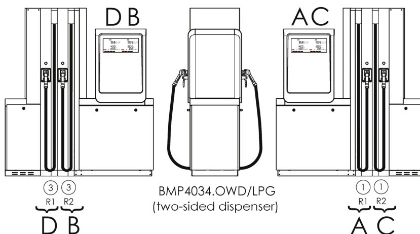
Image 22 – Exemple d'appareil distributeur combiné avec quatre points de distribution A, B, C et D (quatre pompages simultanés, quatre écrans principaux; ①, ②, ③ ... - position de la buse dans la calculatrice)
