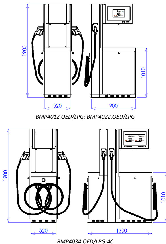
Image 5 - Aperçu des modèles standards d'appareils distributeurs OCEAN EURO GPL sans enrouleurs de flexibles
