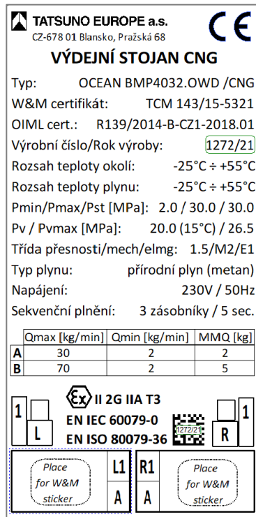
Obrázek 64 - Typový štítek dvou hadicového stojanu CNG
