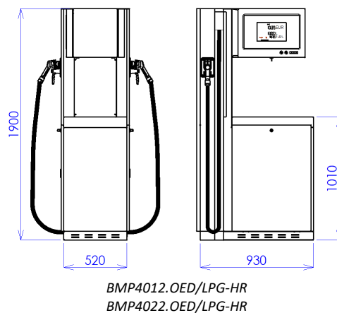
Obrázek 17 - Standardní model stojanu OCEAN EURO LPG s navijáky výdejních hadic
