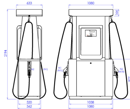
BMP4012.OHD-S; BMP4022.OHD-S
