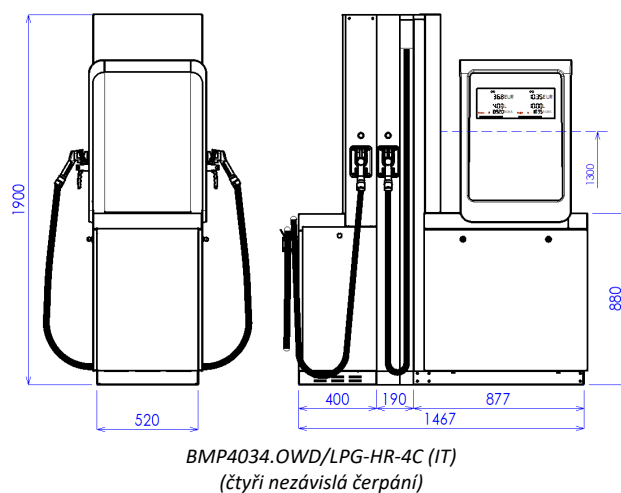
Obrázek 31 – Speciální italská varianta stojanu OCEAN TOWER LPG se dvěma navijáky výdejních hadic a dvěma volně visícími hadicemi (pro delší dosah výdejní pistole)
