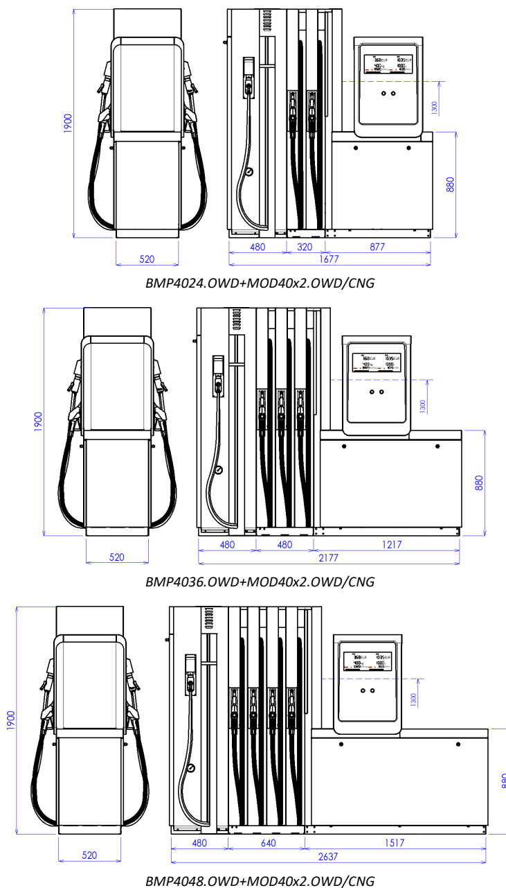
Obrázek 44 - Přehled standardních modelů stojanu OCEAN TOWER COMBI CNG v základním provedení, x=1,2,3 je počet CNG vstupů
