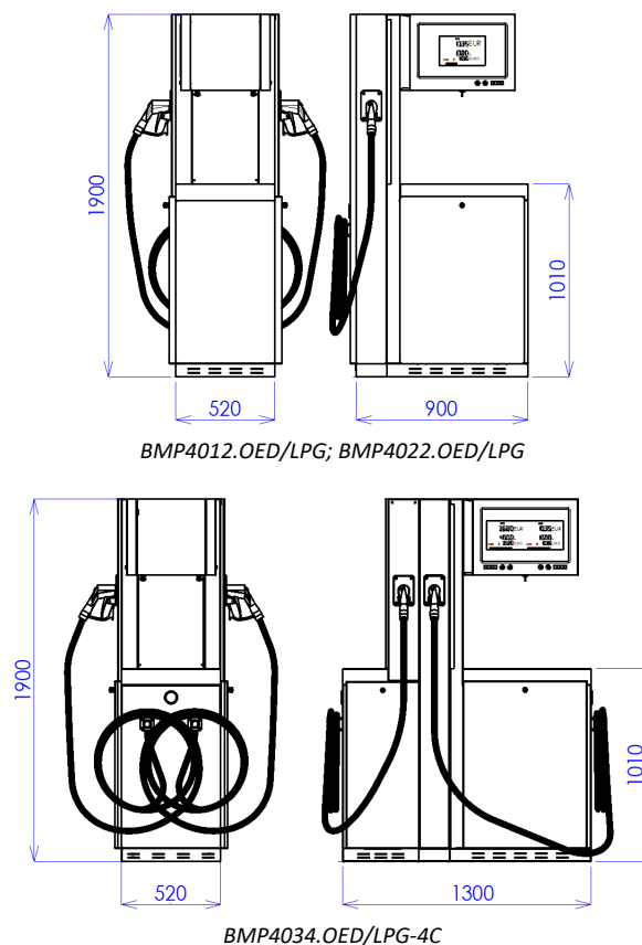
Obrázek 16 - Standardní modely stojanu OCEAN EURO LPG bez navijáků hadic
