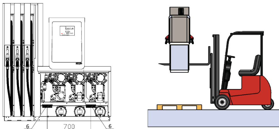
Obrázek 67 – Vyzdvížení stojanu z dřevěné přepravní palety
