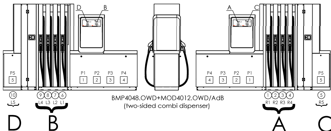
Obrázek 82 – Příklad kombinovaného výdejního stojanu se čtyřmi výdejními místy A, B, C a D (čtyři současně výdeje, čtyři hlavní displeje; ①, ②, ③ ... - pozice hadic v počítadle)
