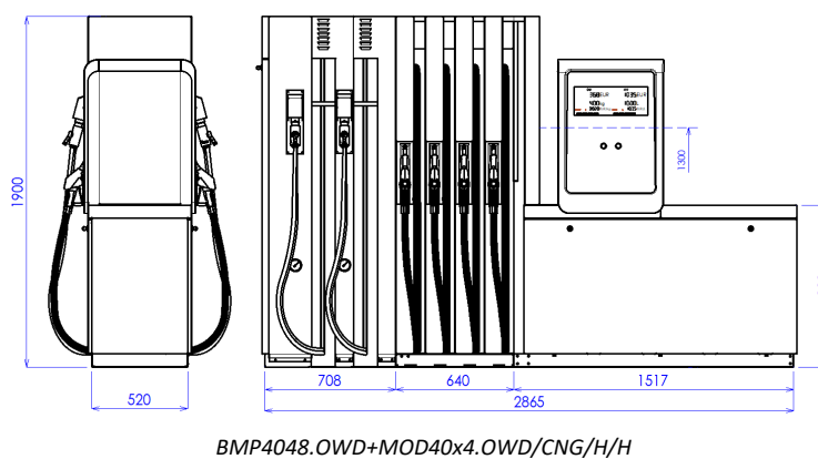
Obrázek 45 – Příklad modelu stojanu OCEAN TOWER COMBI CNG se dvěma výdejními hadicemi CNG na standardní a vysoký výkon (/H)
