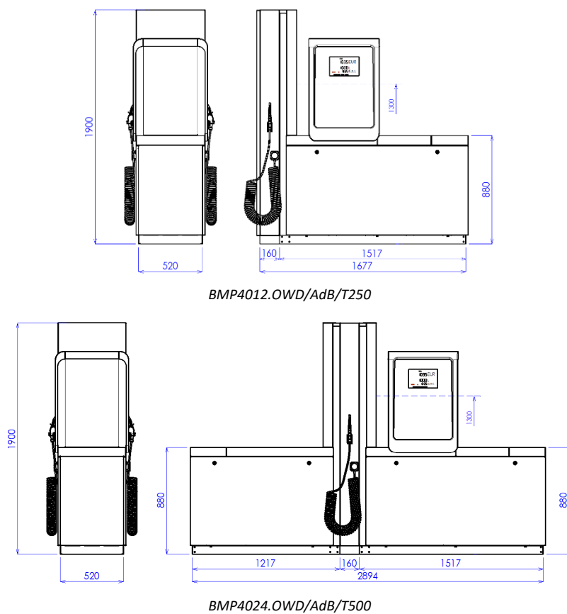
Obrázek 37 – Speciální modely stojanu OCEAN TOWER WSE se sacím čerpadlem zásobní nádrží na 250L nebo 500L média
