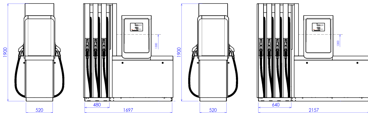
BMP4036.OWD
