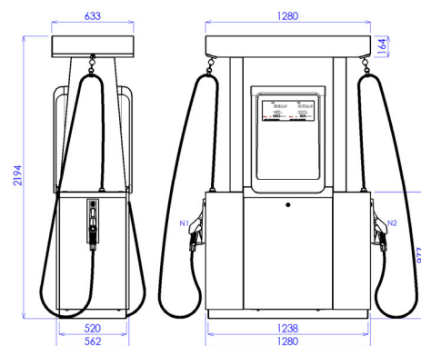
BMP4042.OHD/UH/UH-S
