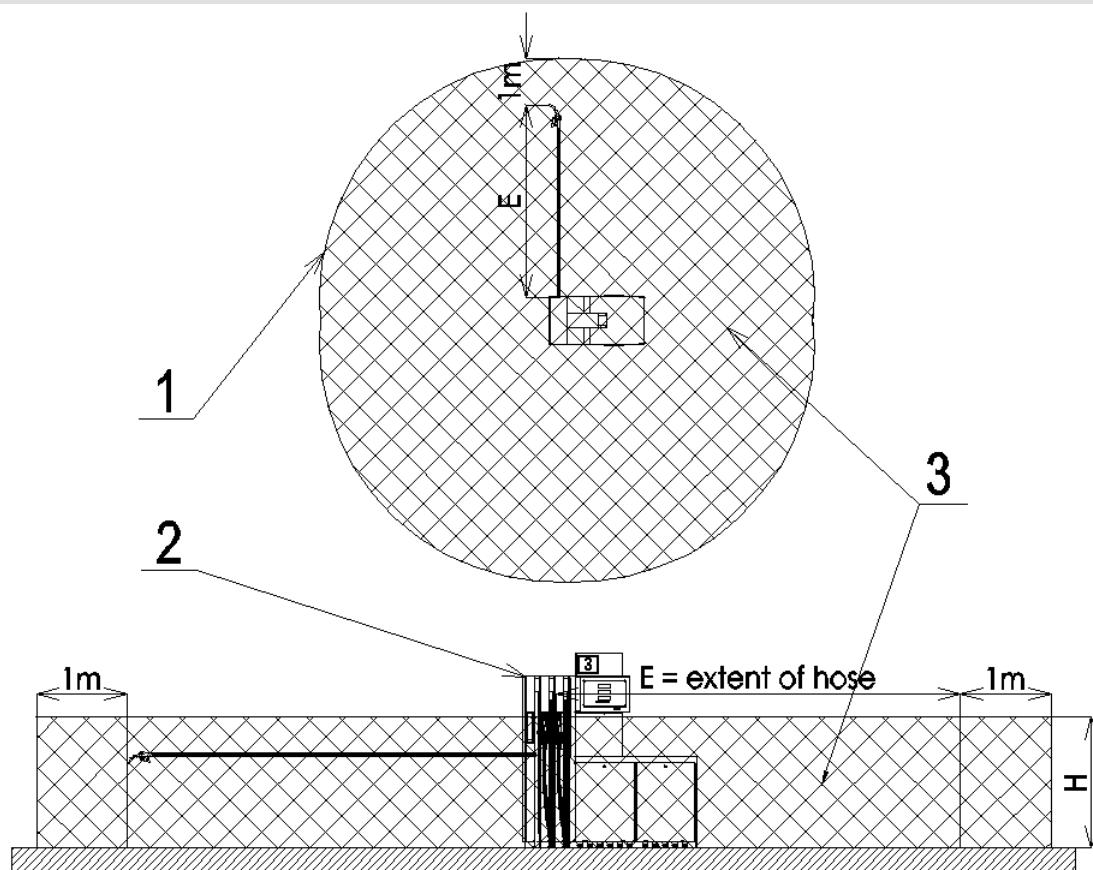
Obrázek 72 - Prostorové omezení pro AdBlue® stojany bez certifikace ATEX
