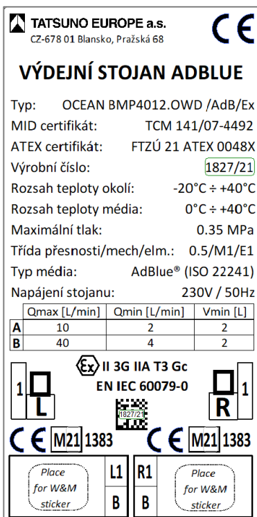
Obrázek 62 - Typový štítek dvou hadicového stojanu AdBlue®
