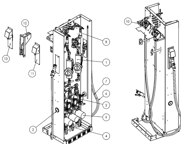
Obrázek 56 - Základní části výdejního modulu WSE a jeho krytování
