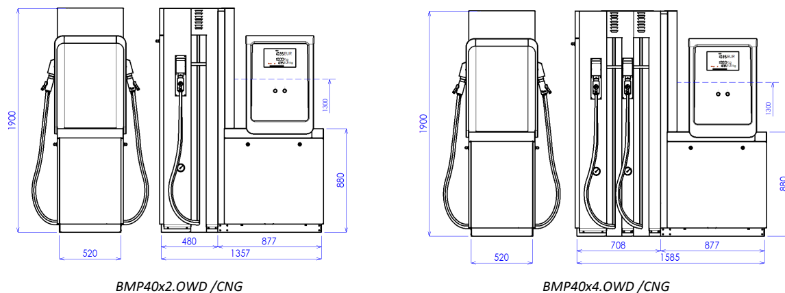
Obrázek 38 – Standardní modely stojanu OCEAN TOWER CNG
