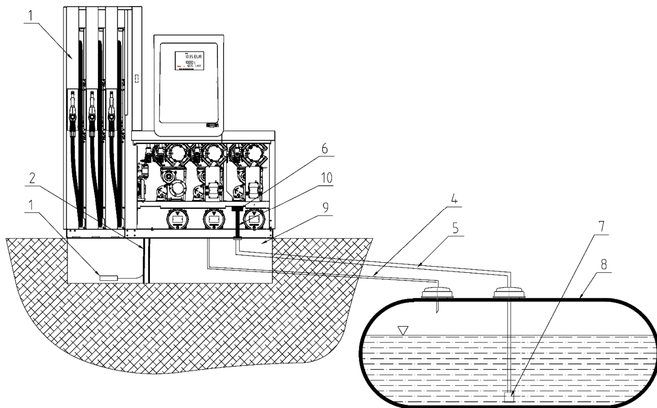
Obrázek 73 - Příklad připojení stojanu se sacími čerpadly k podzemní nádrži
