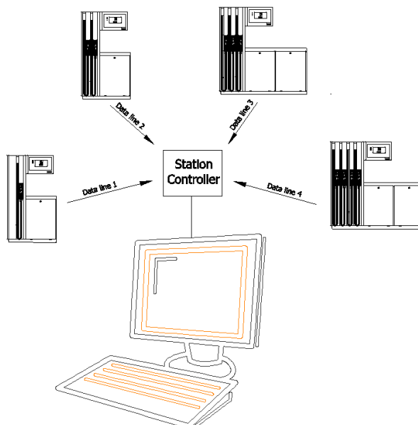
Obrázek 78 - Paprskovité vedení datových linek od stojanů
