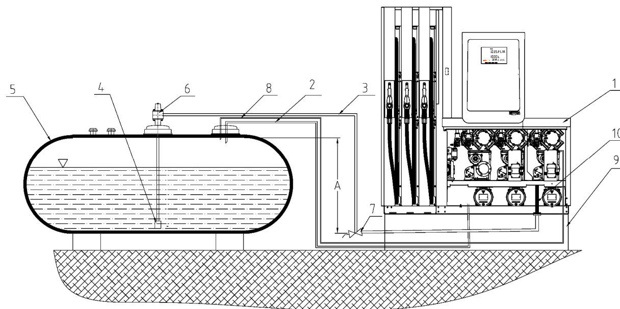
Obrázek 74 - Příklad připojení stojanu se sacími čerpadly k nadzemní nádrži
