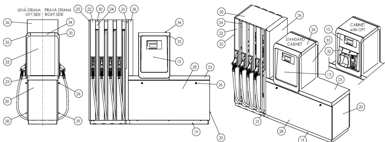
Obrázek 52 - Krytování výdejního stojanu OCEAN TOWER
