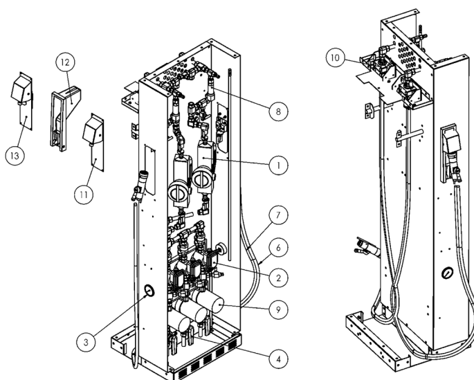
Obrázek 56 - Základní části výdejního modulu WSE a jeho krytování
