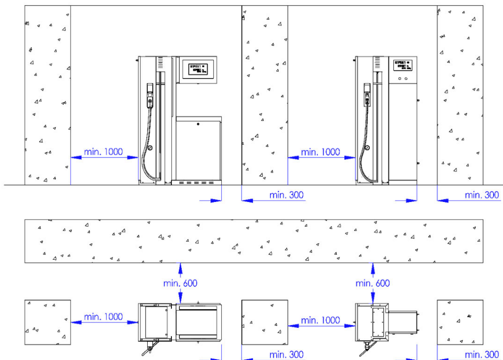
Obrázek 68 – Doporučené minimální vzdálenosti stojanu od pevné překážky
