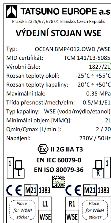
Obrázek 63 - Typový štítek dvou hadicového stojanu WSE
