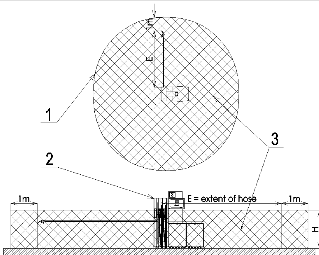
Obrázek 72 - Prostorové omezení pro AdBlue® stojany bez certifikace ATEX
