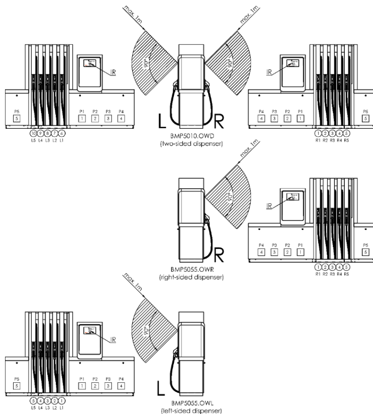
Obrázek 79 - Dosah činnosti dálkového ovladače a značení hadic a produktů výdejního stojanu v elektronickém počítadle (IR – pozice infra červeného přijímače na displeji; ; ①, ②, ③ ... - pozice hadic v počítadle)
