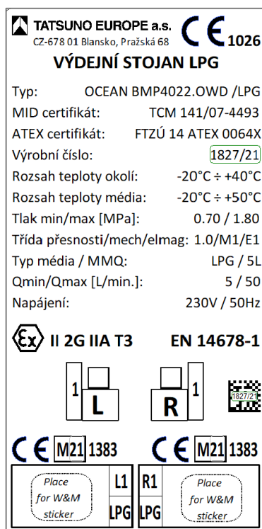
Obrázek 61 - Typový štítek dvou hadicového stojanu LPG
