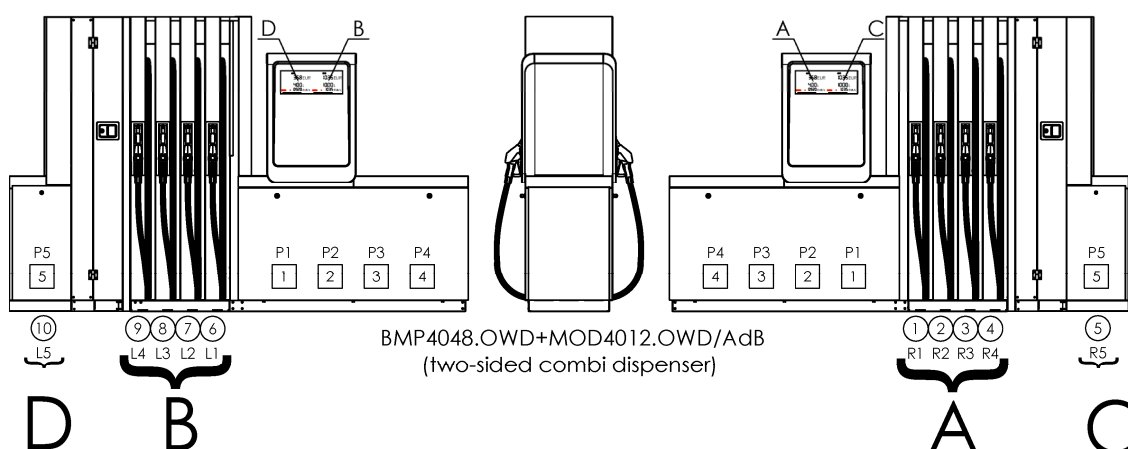
Obrázek 82 – Příklad kombinovaného výdejního stojanu se čtyřmi výdejními místy A, B, C a D (čtyři současně výdeje, čtyři hlavní displeje; ①, ②, ③ ... - pozice hadic v počítadle)
