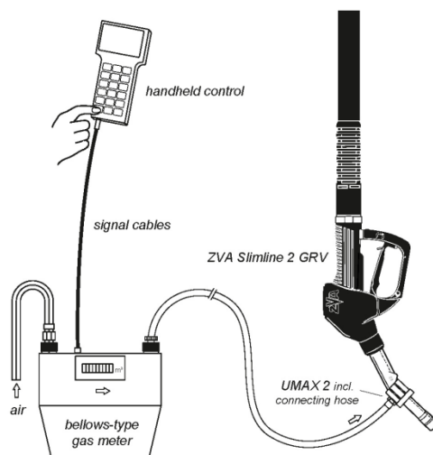
Obrázek 84 – Propojení výdejní pistole s adaptérem a plynoměrem
