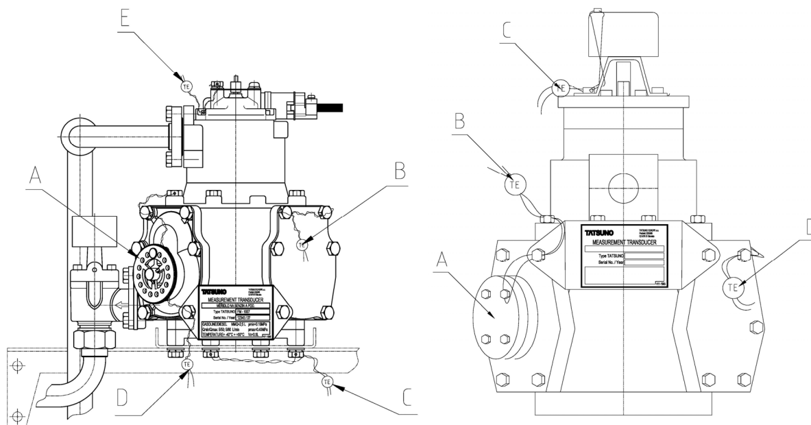
Obrázek 92 – Pístové měřiče PHM (typ FM-1007) a LPG (typ MP-02524 a FM-1029), A=kalibrační kolečko
