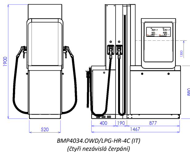
Obrázek 31 – Speciální italská varianta stojanu OCEAN TOWER LPG se dvěma navijáky výdejních hadic a dvěma volně visícími hadicemi (pro delší dosah výdejní pistole)
