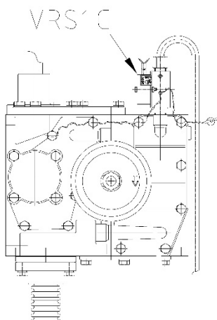
Obrázek 86 - Čerpací monoblok FP-1001 s čidlem odlučování vzduchu VRS1.G
