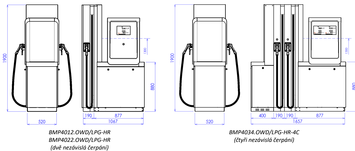
Obrázek 30 - Standardní model stojanu OCEAN TOWER LPG s navijáky výdejních hadic
