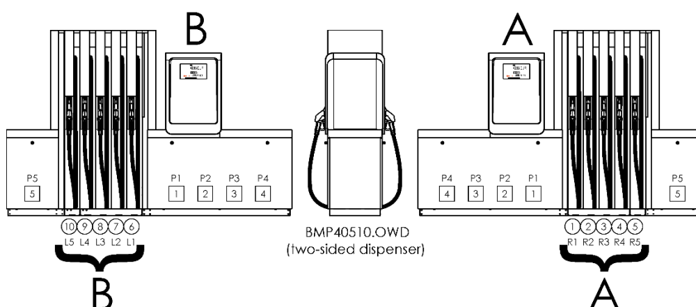
Obrázek 81 – Příklad standardního výdejního stojanu se dvěma výdejními místy A a B (dva současně výdeje, dva hlavní displeje; ①, ②, ③ ... - pozice hadic v počítadle)
