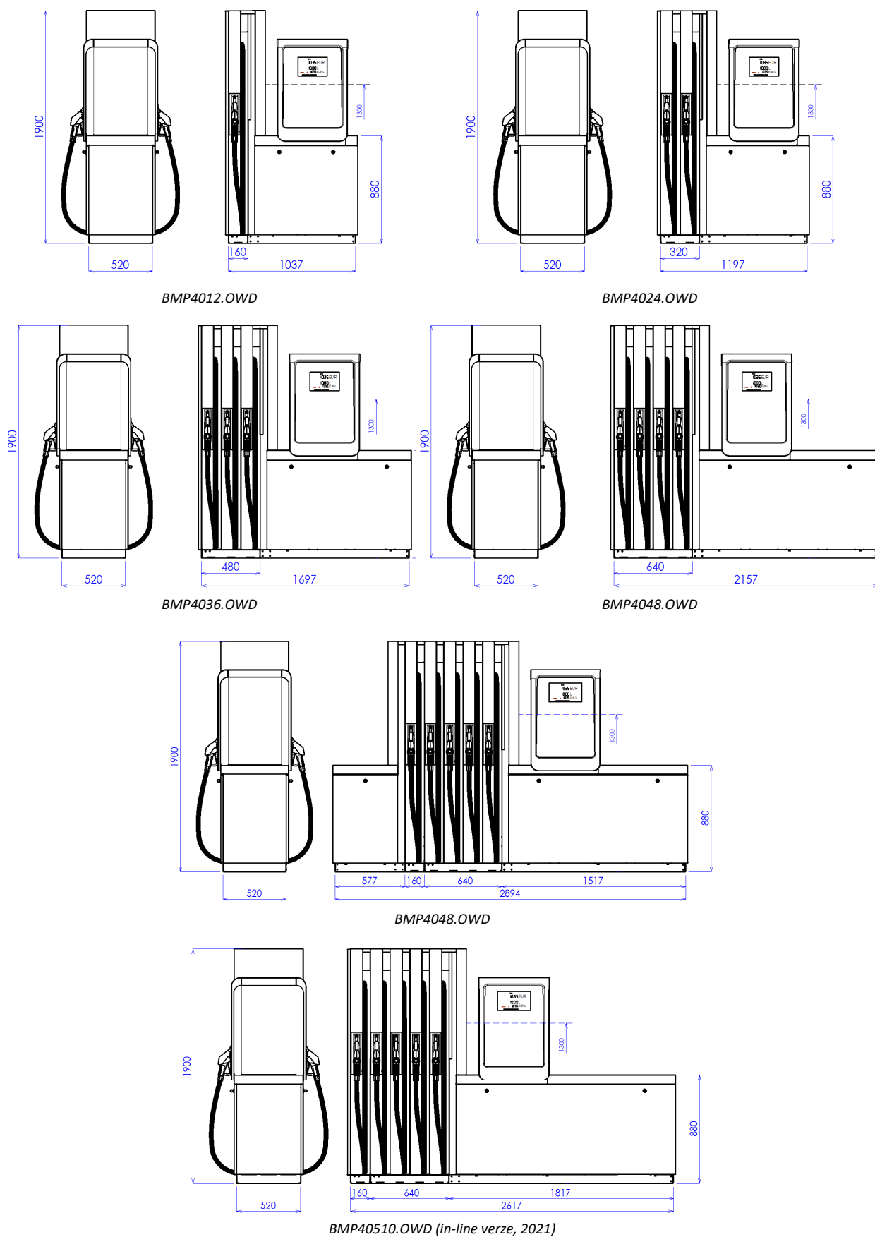
Obrázek 28 - Standardní modely stojanu OCEAN TOWER v základním provedení
