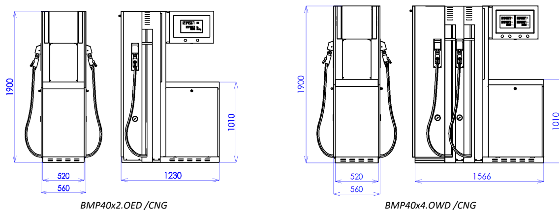
Obrázek 24 – Standardní modely stojanu OCEAN EURO CNG v základním provedení
