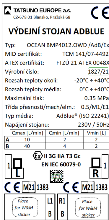
Obrázek 62 - Typový štítek dvou hadicového stojanu AdBlue®
