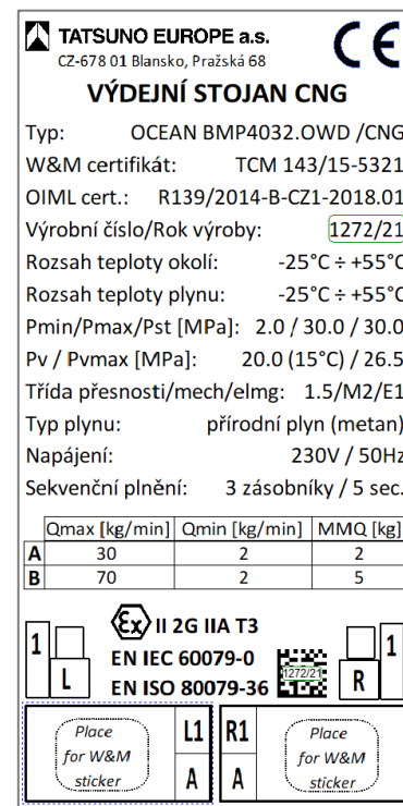
Obrázek 64 - Typový štítek dvou hadicového stojanu CNG
