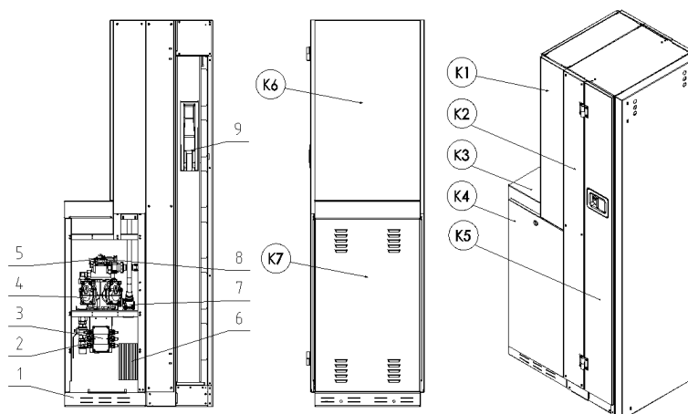
Obrázek 54 - Základní části výdejního modulu AdBlue® a jeho krytování
