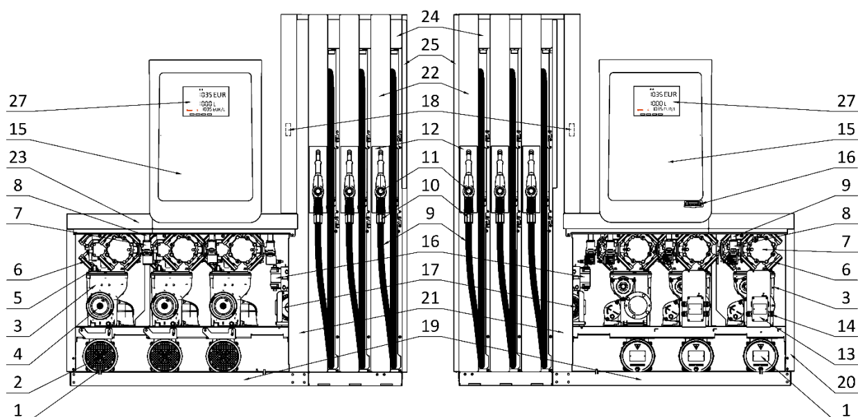
Obrázek 51 - Základní části výdejního stojanu OCEAN TOWER
