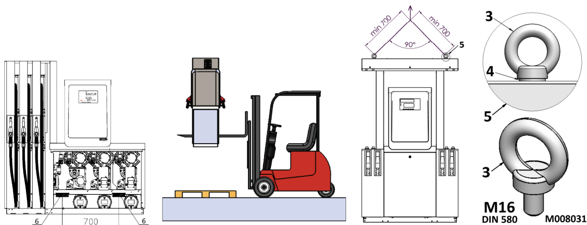
Obrázek 67 – Vyzdvižení stojanu z dřevěné přepravní palety
