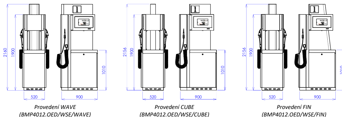
Obrázek 21 – Designové varianty modelů stojanu OCEAN EURO WSE
