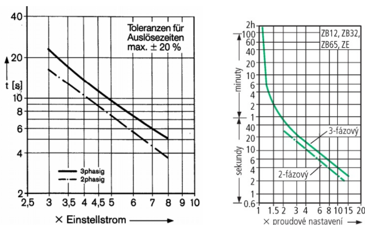
Obrázek 76 - Vybavovací charakteristiky motorové proudové ochrany typu ZE
