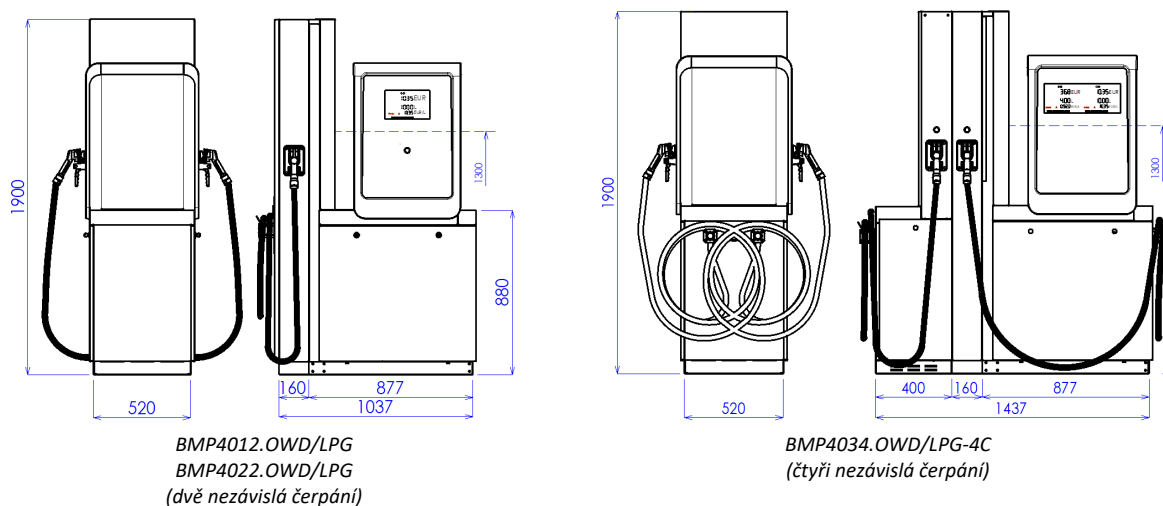
Obrázek 29 – Standardní modely stojanu OCEAN TOWER LPG s volně visícími hadicemi
