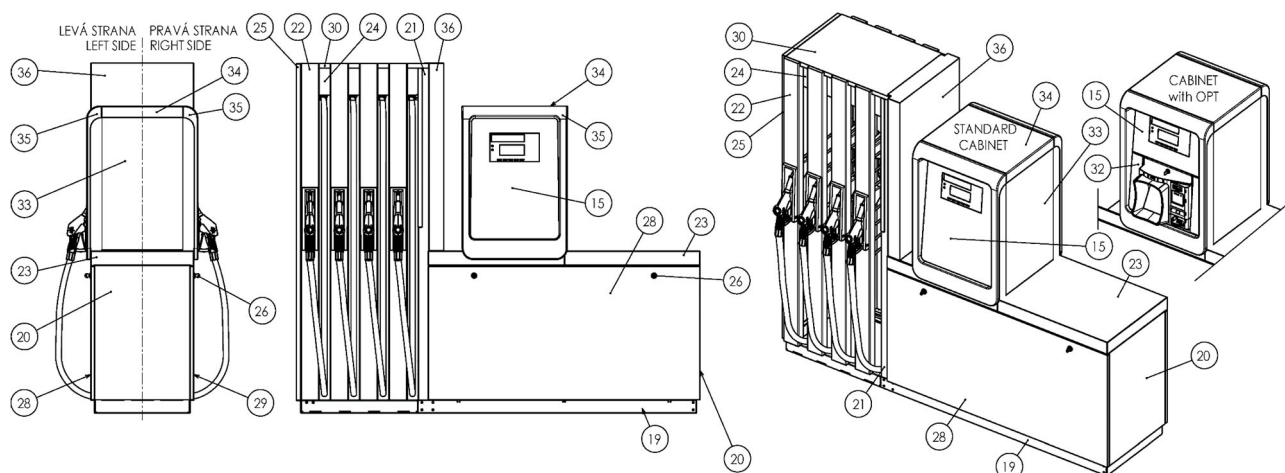
Obrázek 55 - Krytování výdejního stojanu OCEAN TOWER
