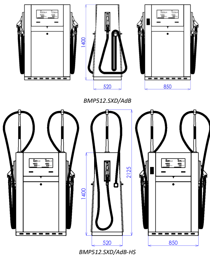
Obrázek 10 - Standardní modely stojanů SHARK ECONOMY ADBLUE® (dvě současná čerpání)
