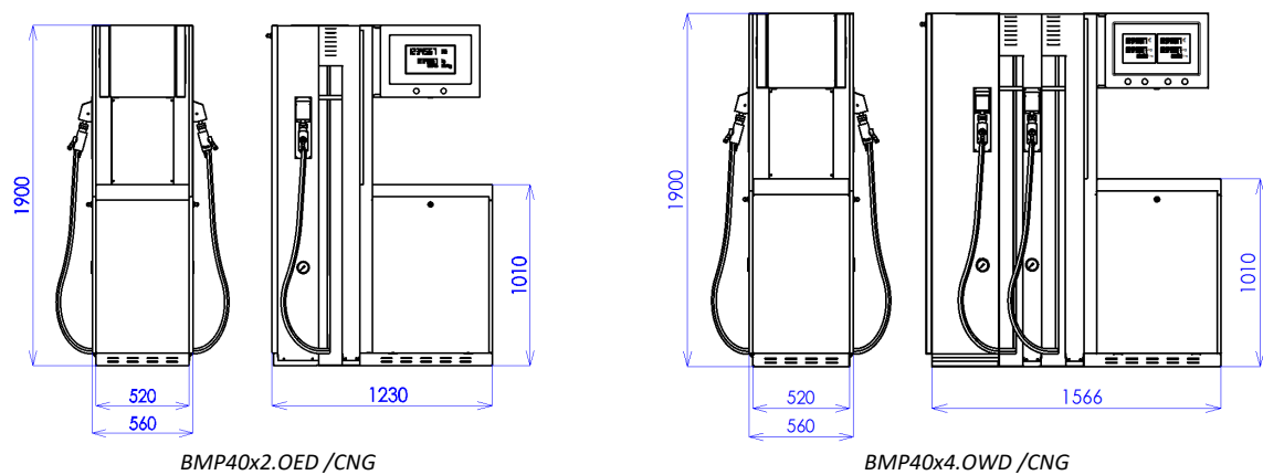
Obrázek 27 – Standardní modely stojanu OCEAN EURO CNG v základním provedení
