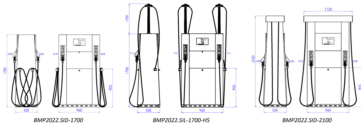
Obrázek 14 - Standardní modely stojanů SHARK ISLAND – hadice z čela
