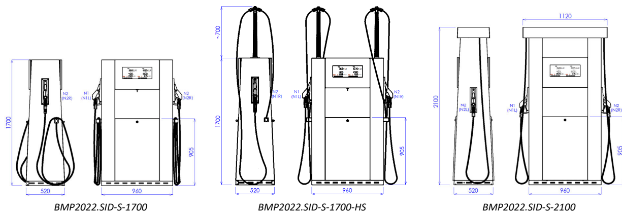
Obrázek 13 - Standardní modely stojanů SHARK ISLAND - hadice z boku (-S)
