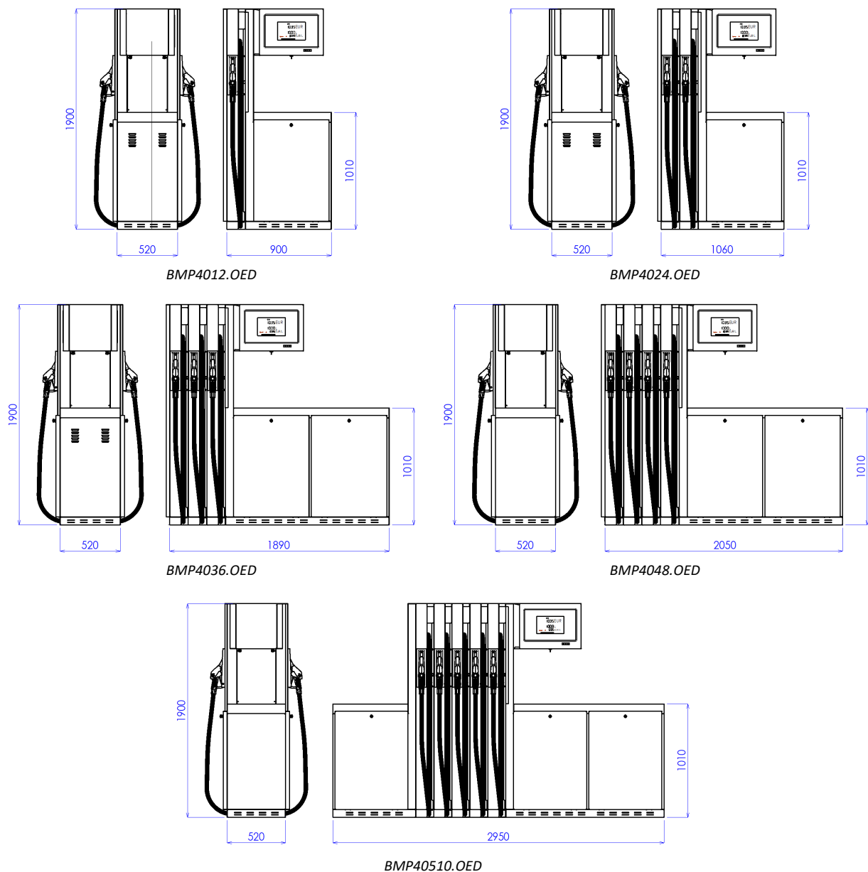
Obrázek 16 - Standardní modely stojanu OCEAN EURO v základním provedení
