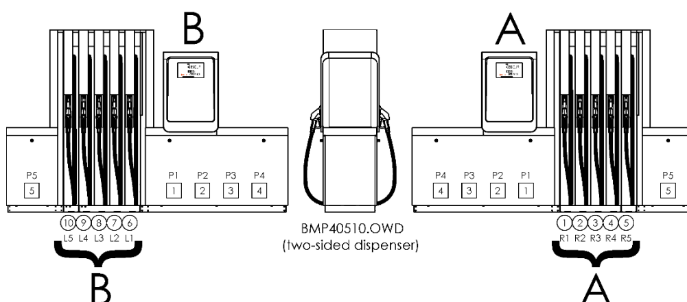
Obrázek 84 – Příklad standardního výdejního stojanu se dvěma výdejními místy A a B (dva současně výdeje, dva hlavní displeje; ①, ②, ③ ... - pozice hadic v počítadle)
