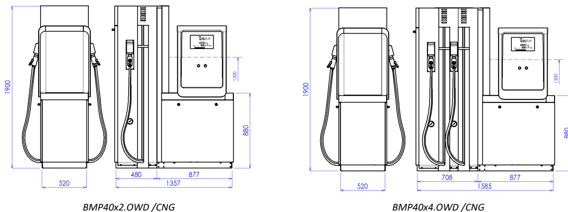
Obrázek 41 – Standardní modely stojanu OCEAN TOWER CNG
