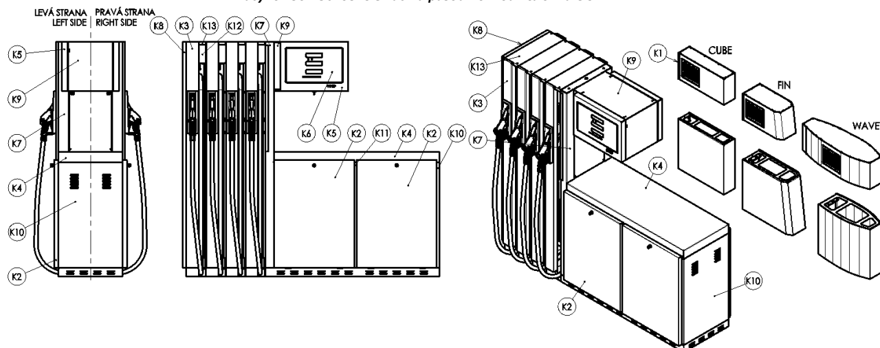
Рисунок 37 - Зачехление раздаточной колонки OCEAN
