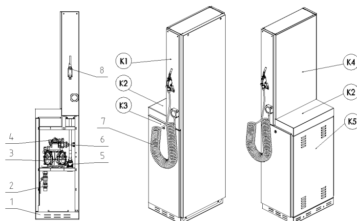
Рисунок 40 - Основные части раздаточного модуля WSE и его зачехления
