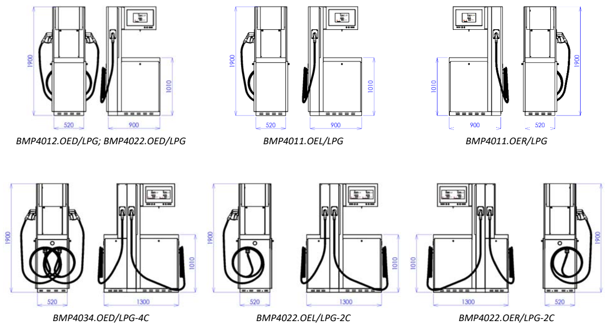
Рисунок 23 - Перечень стандартных моделей колонок OCEAN EURO LPG без намоточного устройства для шлангов
