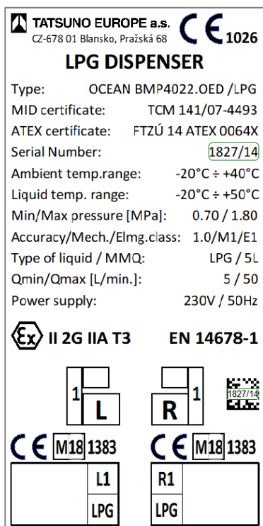
Рисунок 46 - Типовой шильдик колонки с двумя шлангами LPG
