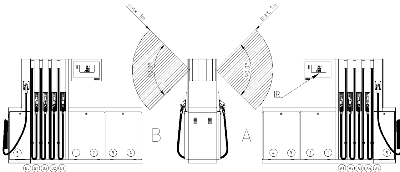
Рисунок 58 - Достижимость действия дистанционного управляющего устройства и обозначение шлангов, а также продуктов раздаточной колонки
