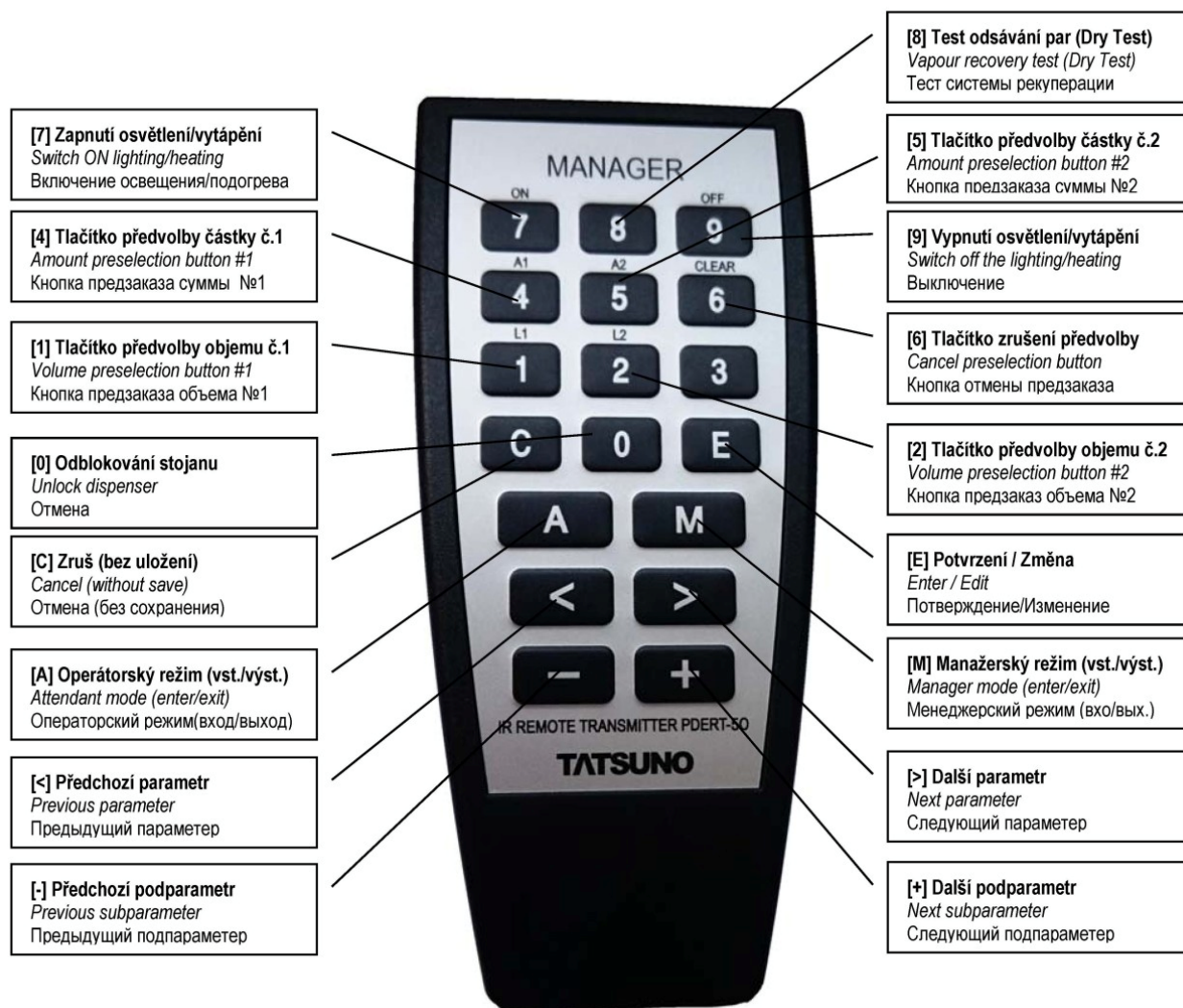
Рисунок 59 - Описание кнопок дистанционного управляющего устройства PDERT-50
