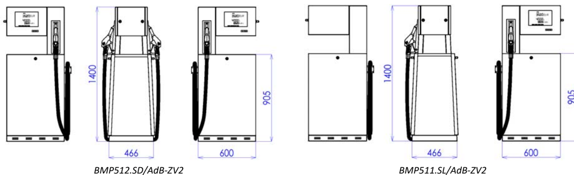
Рисунок 7 - Стандартные модели колонок SHARK JUNIOR ADBLUE® с пистолетами на передней панели (-ZV2)
