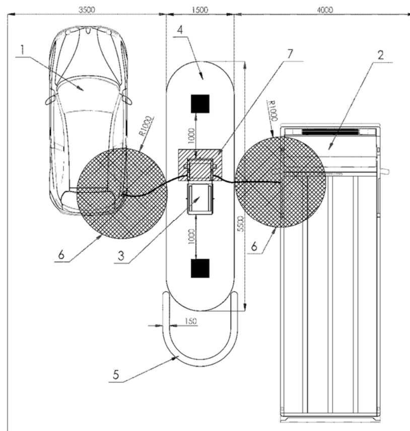
Рисунок 51 – Пример размещения раздаточной колонки CNG на заправочной станции
