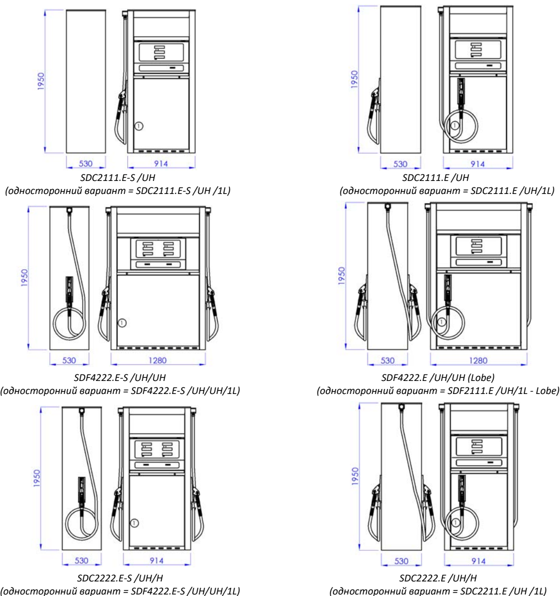
Рисунок 17 - Модели колонок SUNNY-XE EURO для выдачи дизеля в больших объемах
