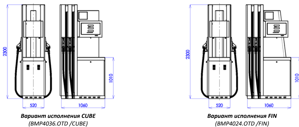
Рисунок 19 – Дизайнерские варианты моделей колонок OCEAN TALL
