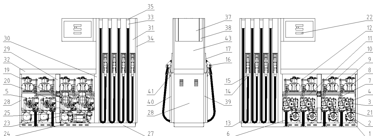
Рисунок 36 - Основные части раздаточной колонки OCEAN
