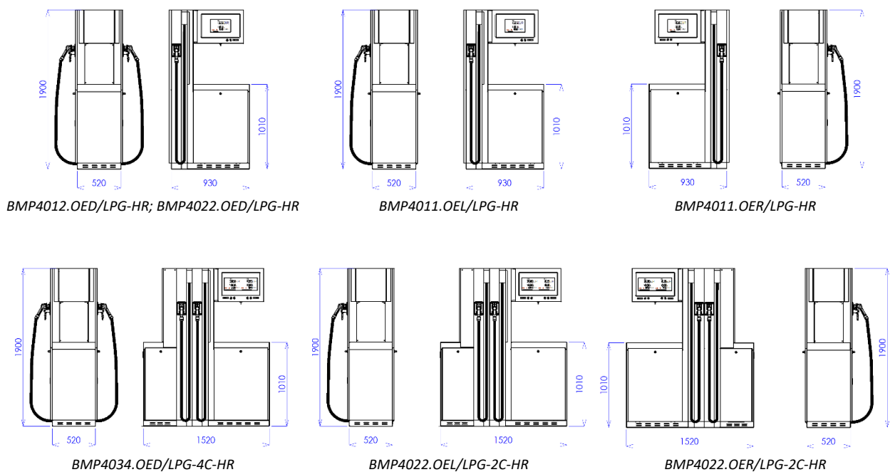
Рисунок 24 - Перечень стандартных моделей колонок OCEAN EURO LPG с намоточным устройством для шлангов
