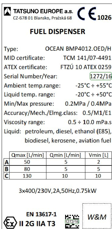
Рисунок 43 - Типовой шильдик колонки бензин/дизель с несколькими шлангами
