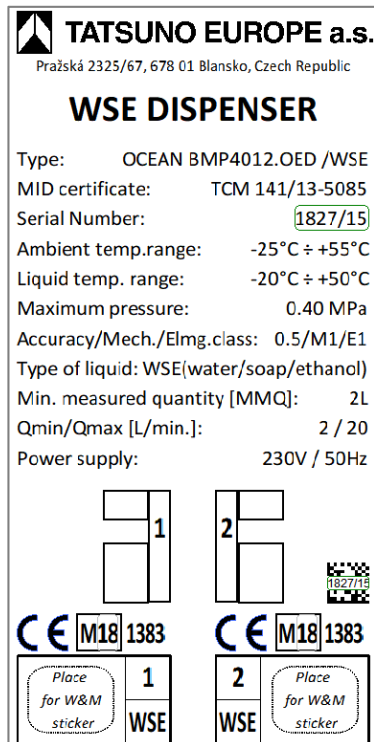
Рисунок 48 - Типовой шильдик колонки с двумя шлангами WSE
