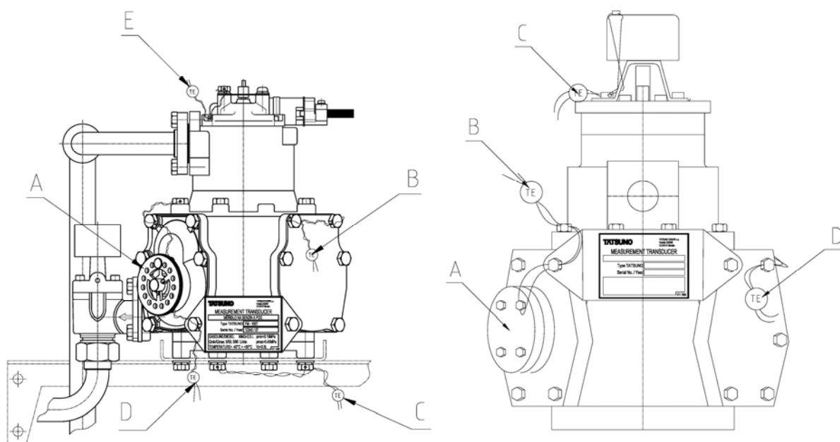
Рисунок 66 – Поршневые измерители топлива (тип FM-1007, FM1025) и LPG (тип MP-02524 и FM-1029), A=калибровочное колесико
