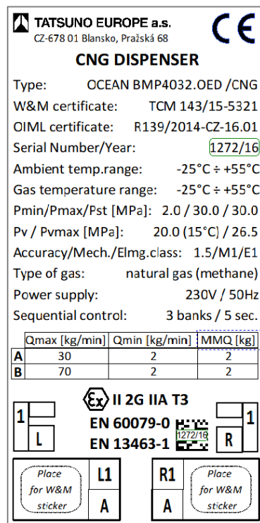
Рисунок 49 - Типовой шильдик колонки с двумя шлангами CNG
