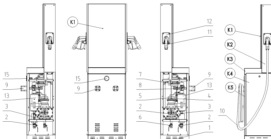
Рисунок 38 - Основные части раздаточного модуля LPG и его зачехление
