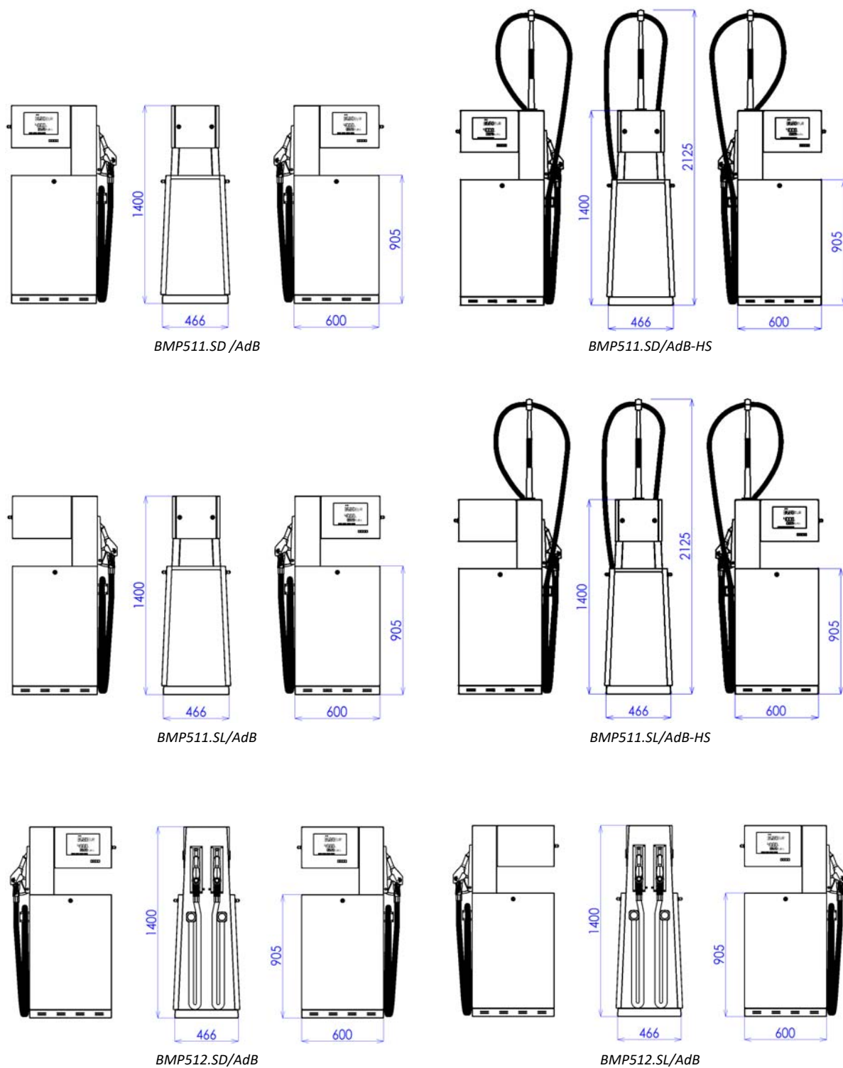
Рисунок 8 - Стандартные модели колонок SHARK JUNIOR ADBLUE® с пистолетами, размещенными сбоку
