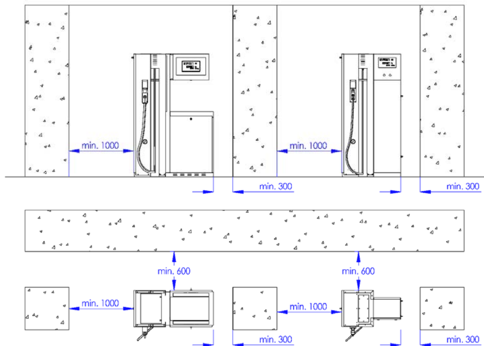
Рисунок 50 – Минимальные расстояния колонки от стационарного препятствия
