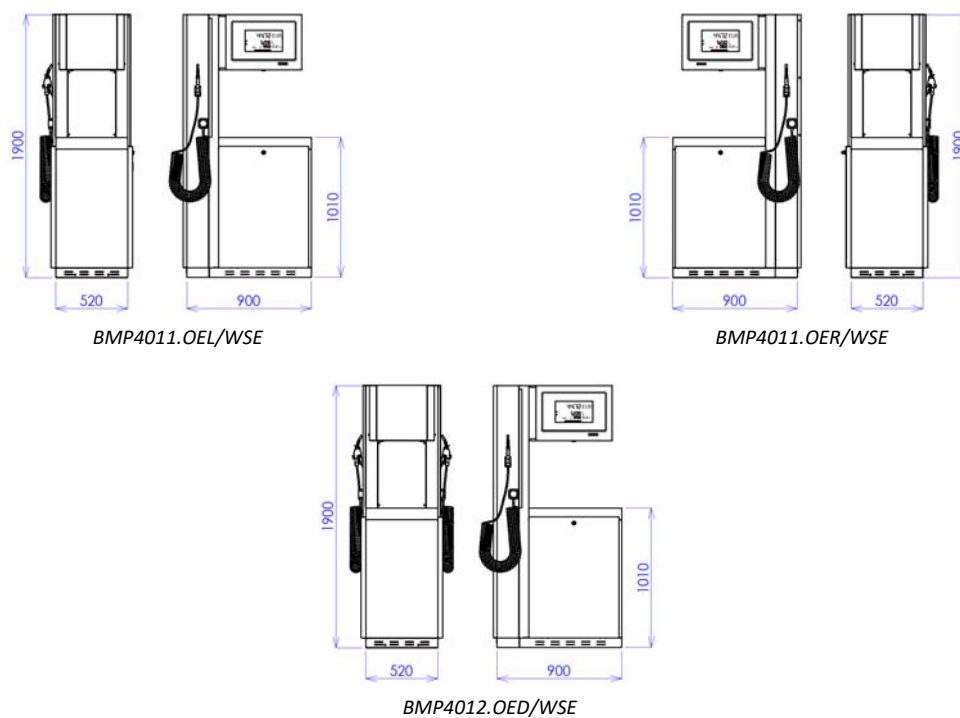
Рисунок 29 - Перечень стандартных моделей колонок OCEAN EURO WSE
