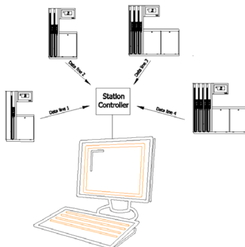
Рисунок 57 - Радиальное расхождение линий передачи данных от колонок
