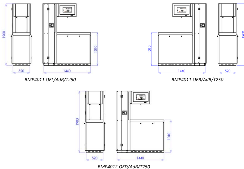
Рисунок 27 - Перечень моделей колонок OCEAN EURO ADBLUE® с резервной емкостью 250 л и насосом
