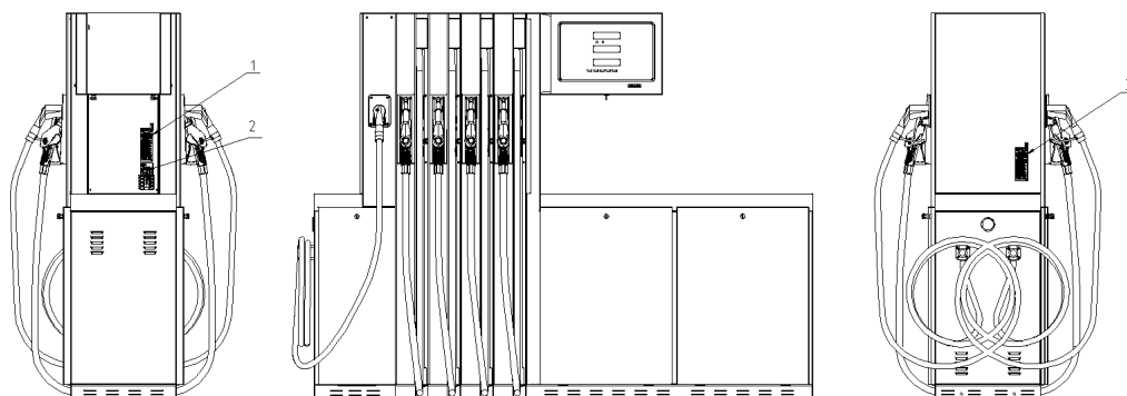
Рисунок 45 - Размещение шильдиков производителя на комбинированной колонке (1 – типовой шильдик бензин / дизель; 2 – ориентировочный шильдик, 3 – типовой шильдик LPG)
