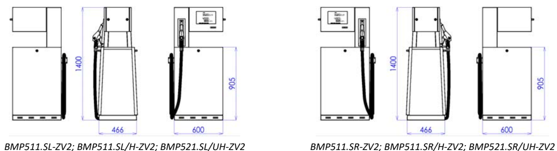
Рисунок 4 - Стандартные модели колонок SHARK JUNIOR с пистолетами на передней панели
