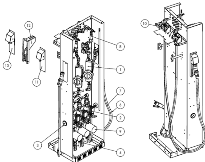
Рисунок 41 - Основные части раздаточного модуля WSE и его зачехления
