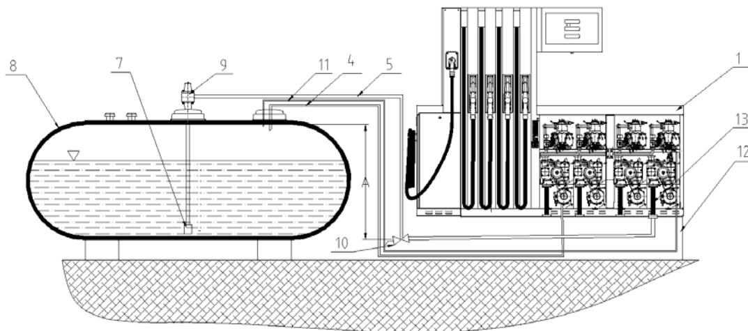
Рисунок 53 - Пример присоединения колонки с всасывающими насосами к наземной емкости
