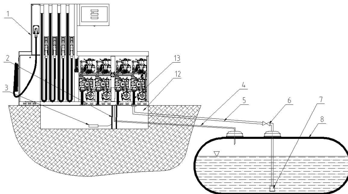
Рисунок 52 - Пример присоединения колонки с всасывающими насосами к подземной емкости
