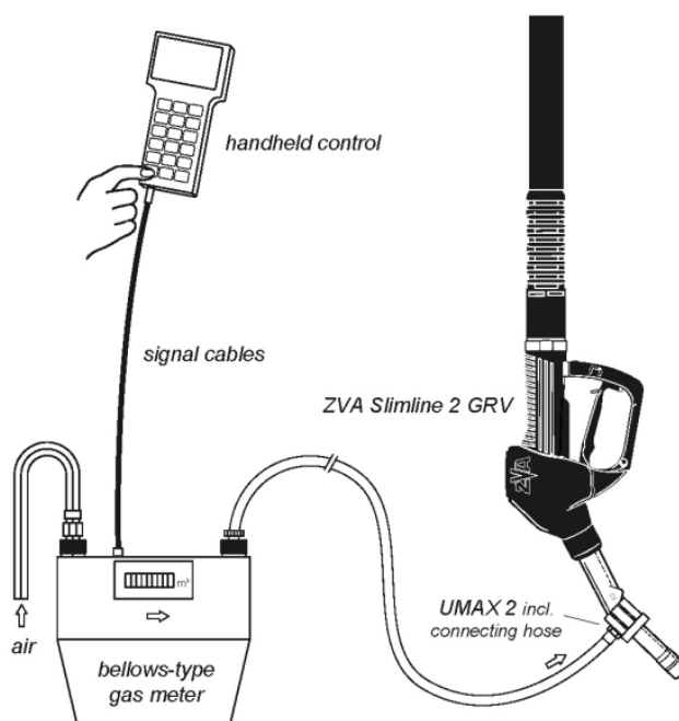
Рисунок 61 – Соединение заправочного пистолета с адаптером и газовым счетчиком
