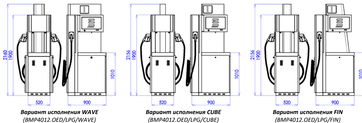
Рисунок 22 – Дизайнерские варианты моделей колонок OCEAN EURO LPG
