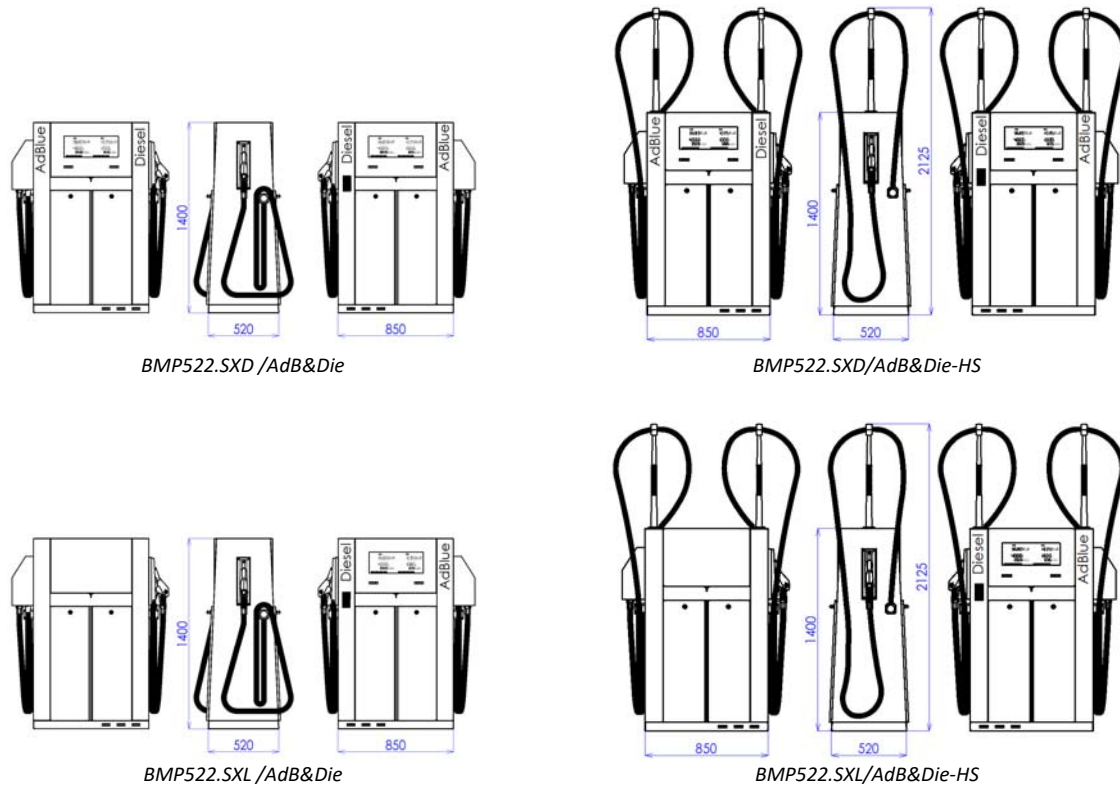
Рисунок 14 - Стандартные модели колонок SHARK ECONOMY COMBI
