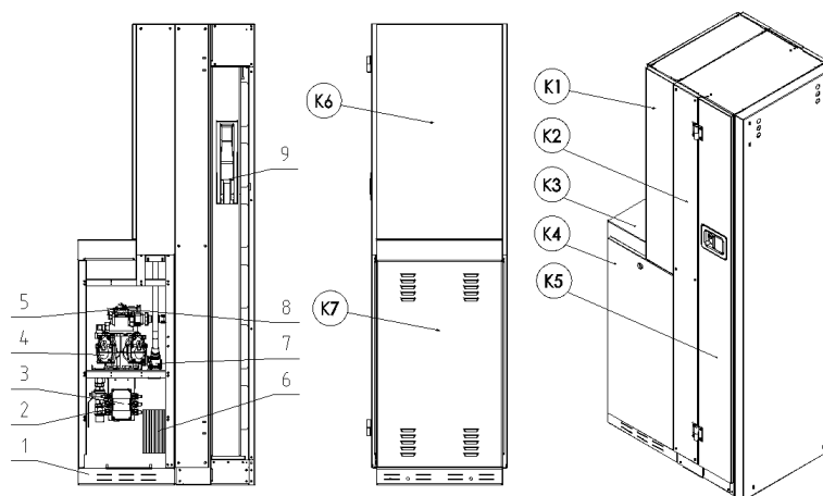
Рисунок 39 - Основные части раздаточного модуля Adblue® и его зачехления
