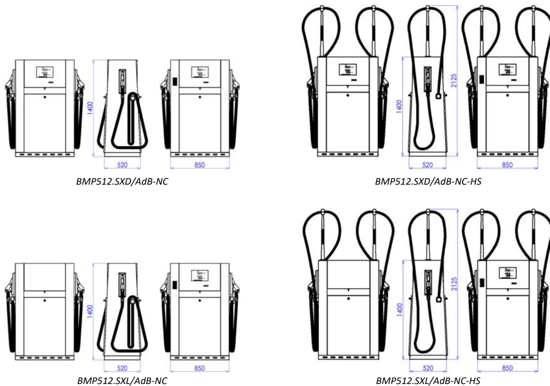
Рисунок 13 - Стандартные модели колонок SHARK ECONOMY ADBLUE® (неодновременные заправки - NC)
