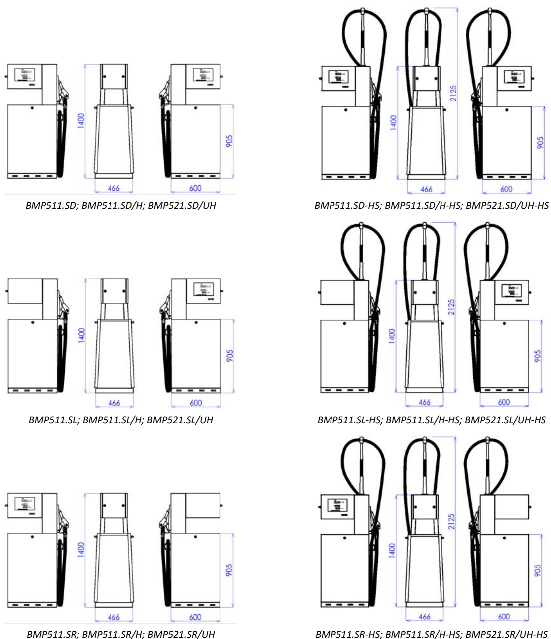
Рисунок 5 - Стандартные модели колонок SHARK JUNIOR с пистолетами сбоку
