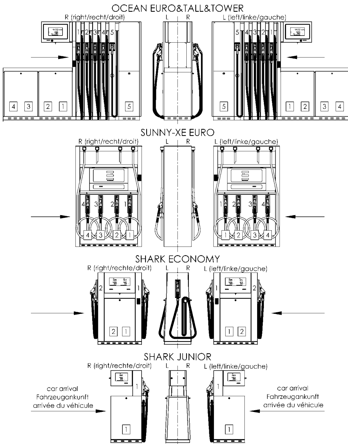
Рисунок 3 - Система обозначений раздаточных колонок с рекомендуемым направлением приезда
