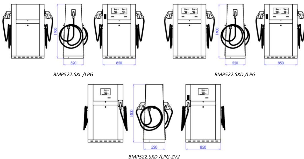
Рисунок 11 - Стандартные модели колонок SHARK ECONOMY LPG
