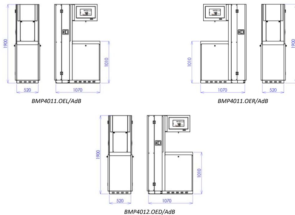
Рисунок 26 - Перечень стандартных моделей колонок OCEAN EURO ADBLUE®
