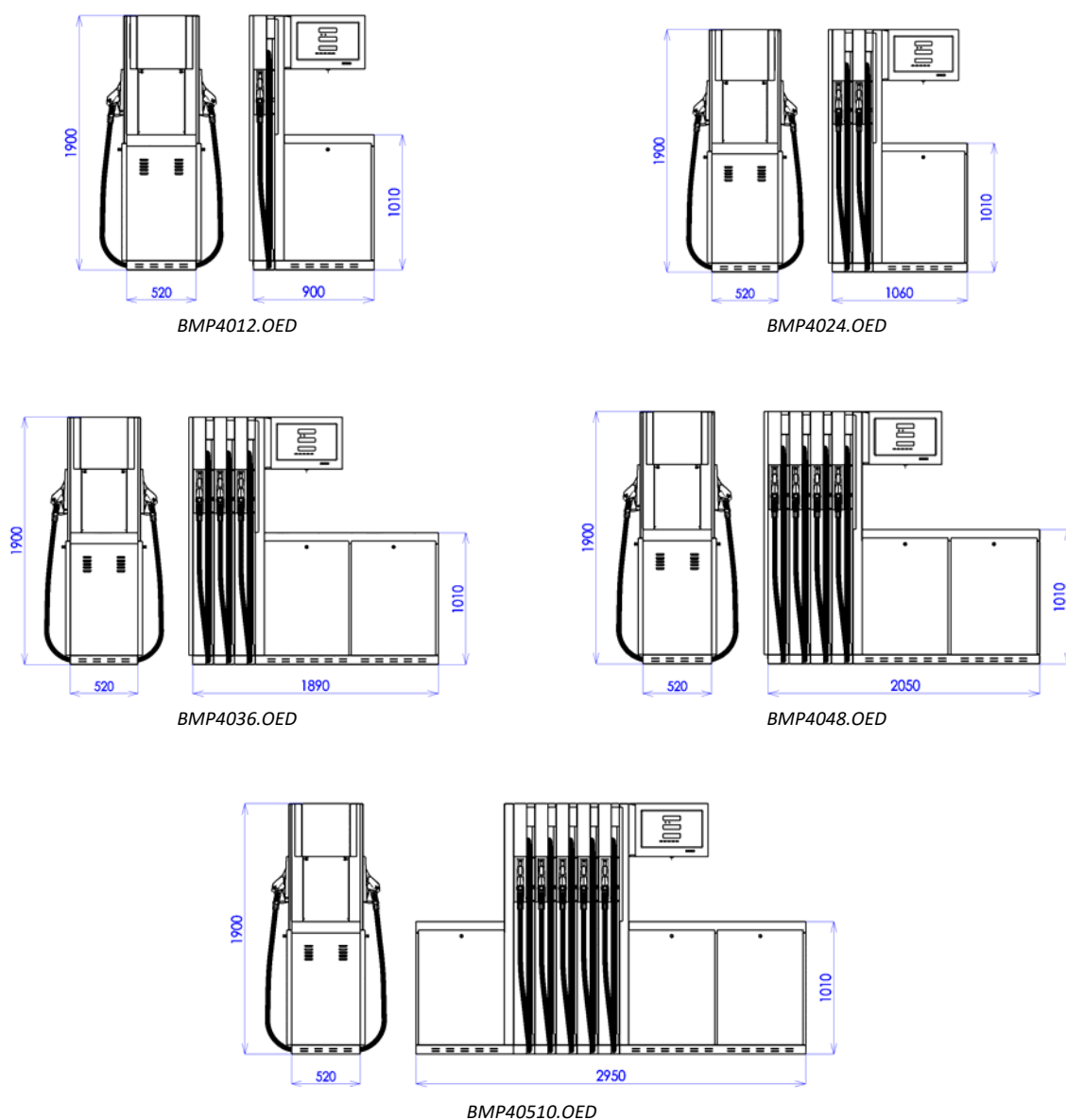
Рисунок 20 - Перечень стандартных моделей колонок OCEAN EURO в базовом варианте исполнения
