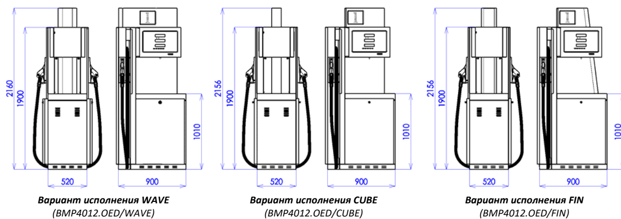
Рисунок 21 – Дизайнерские варианты моделей колонок OCEAN EURO
