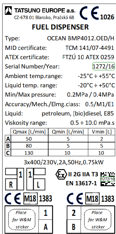
Рисунок 42 - Типовой шильдик колонки бензин / дизель с двумя шлангами
