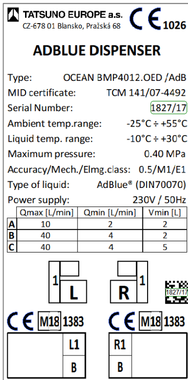
Рисунок 47 - Типовой шильдик колонки с двумя шлангами AdBlue®
