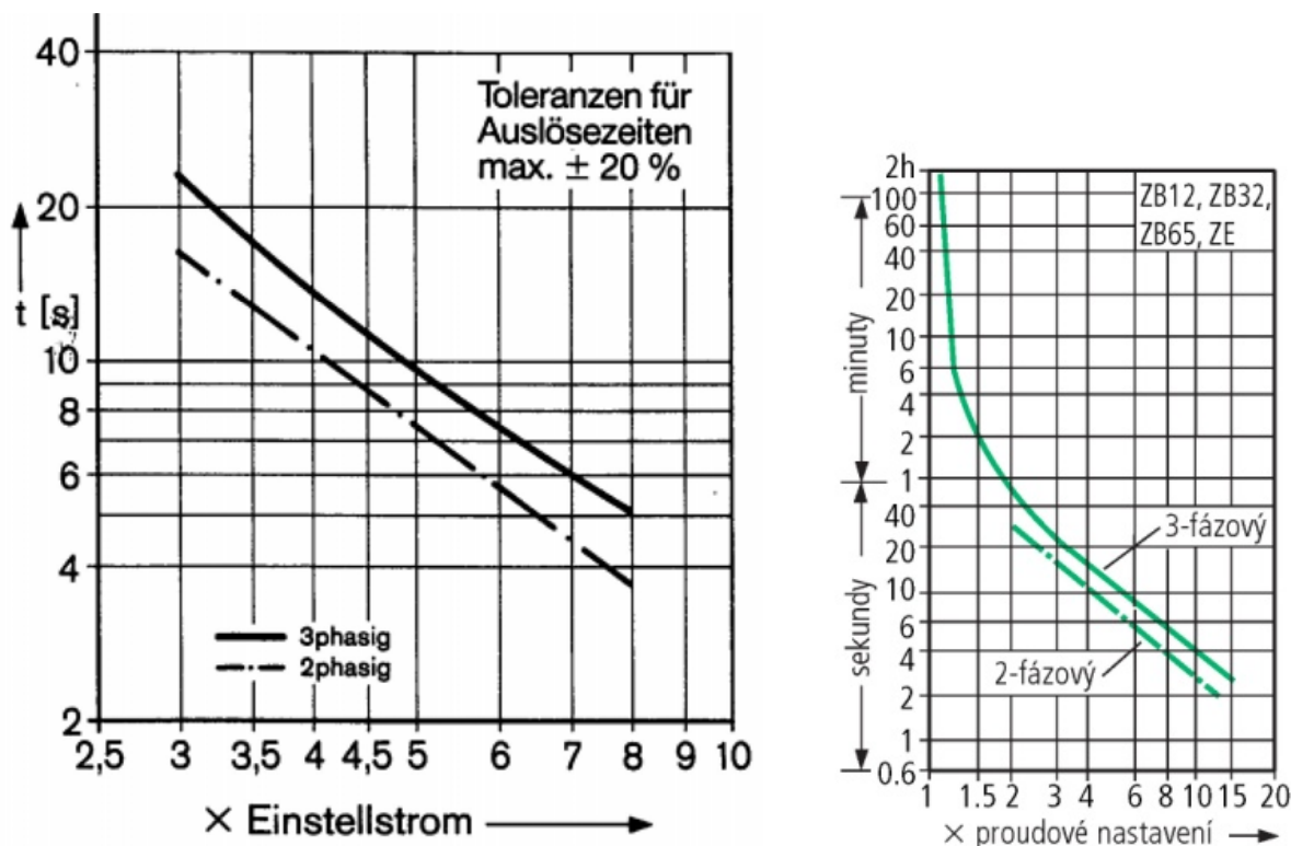
Рисунок 55 - Выборочные характеристики токовой защиты двигателя типа ZE
