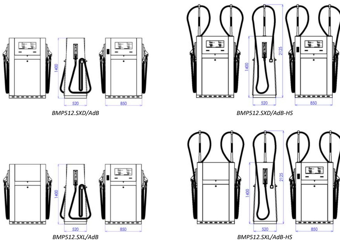
Рисунок 12 - Стандартные модели колонок SHARK ECONOMY ADBLUE® (две одновременные заправки)
