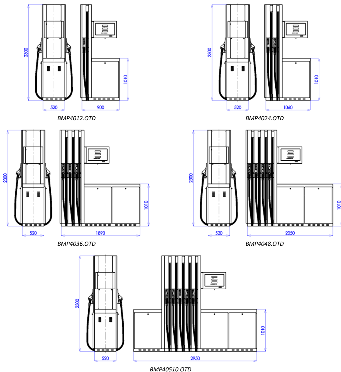
Рисунок 18 - Перечень стандартных моделей колонок OCEAN TALL в базовом варианте исполнения
