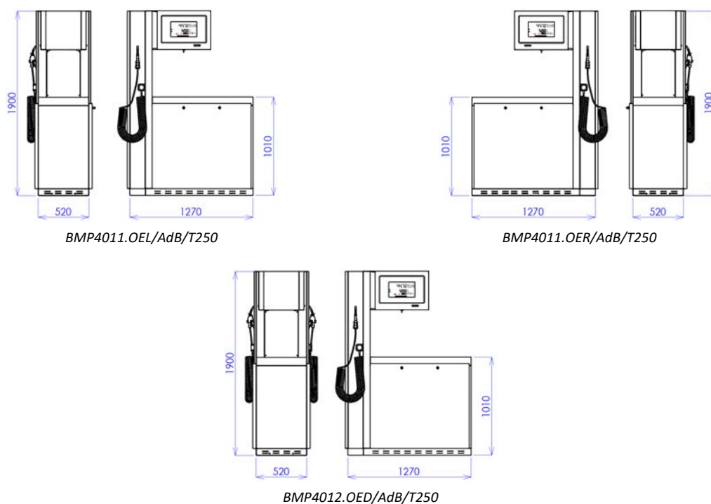
Рисунок 30 - Перечень моделей колонок OCEAN EURO ADBLUE® с резервной емкостью 250 л и насосом
