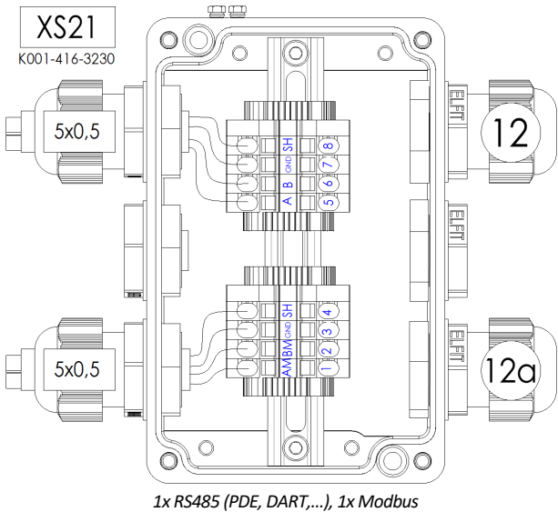
1x RS485 (PDE, DART,...), 1x Modbus
